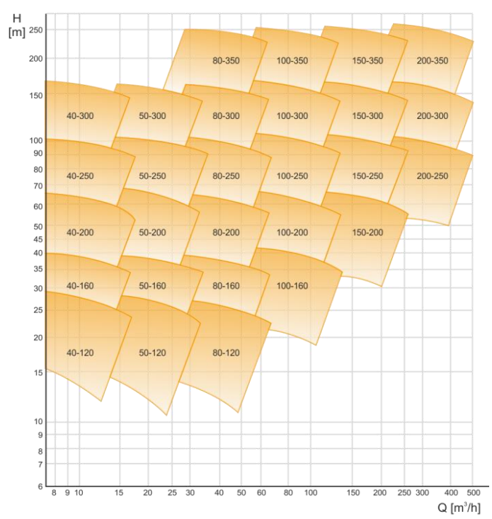
60Hz 3600 RPM
